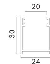
Guida alluminio 30x24 mm con spazzolino 4,8x5
