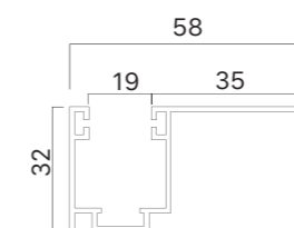
Pretelaio 32x58 mm con spazzolino 4,8x6
