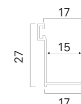
Guida alluminio 27x17 mm con spazzolino 4,8x4
