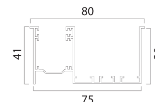
Pretelaio incassata 45 con spazzolino 4,8x6
