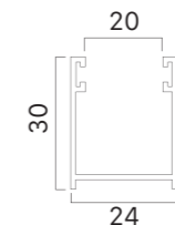
Guida alluminio 30x24 mm con spazzolino 4,8x5
