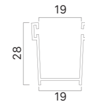
Guida alluminio 28x19 mm con spazzolino 4,8x4
